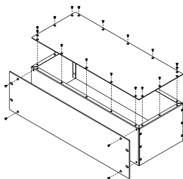
DIN rail enclosures
