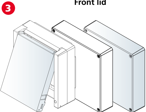
Front lid
